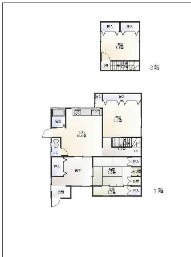
間取図
